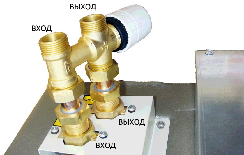
Пример установки 3-х ходового клапана (Вид снизу)
