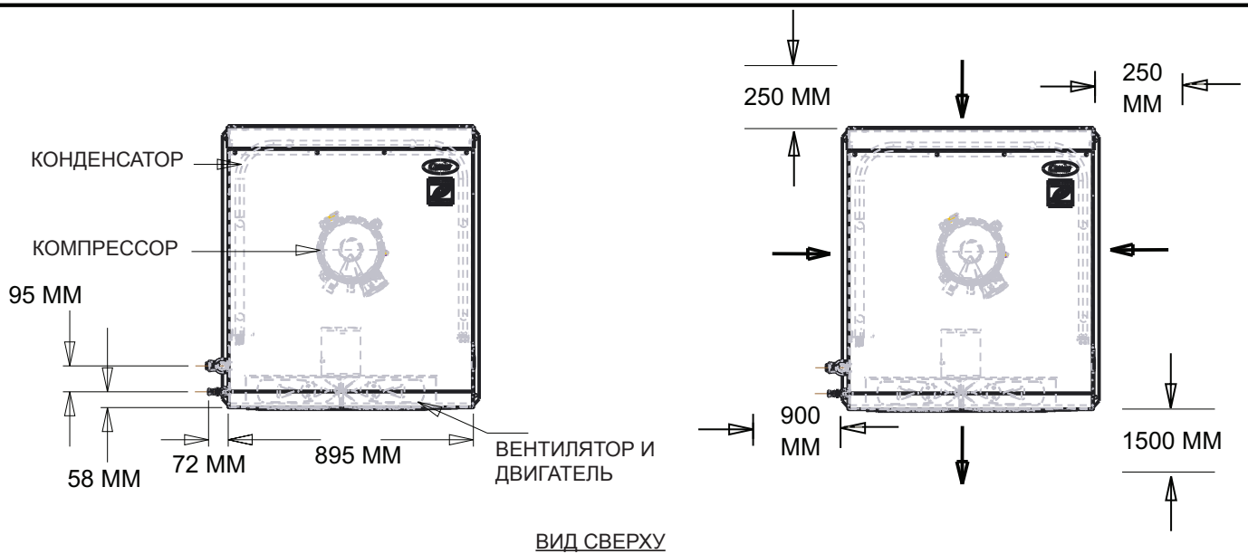
Рис.1 38CMG100/125 Наружный
